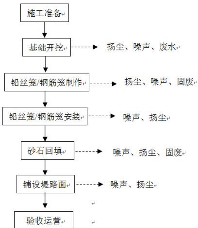
图4-1 项目施工工艺流程及产污节点图
